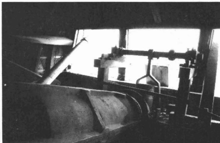
De zware gietijzeren molenas in de rieten kap van de molen in Thesinge..
